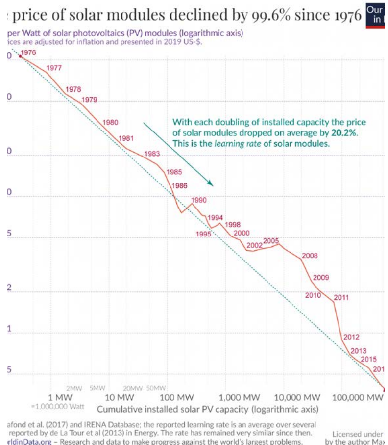
Figuur 5 Kostendaling bij verdubbeling geïnstalleerd volume zon-pv
